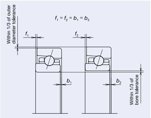
Fig. 3.11 DU Combination
