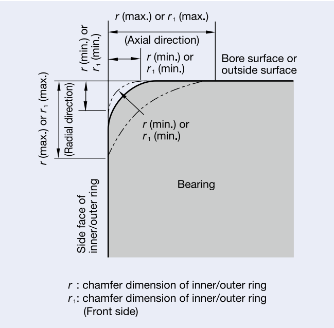
Fig. 8.2 Chamfer Dimension
