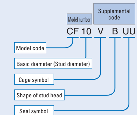
(d) Example of "Basic diameter"
